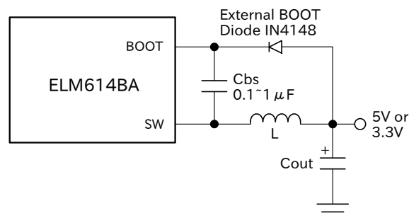
図 2：DCDC コンバータの出力端子から BS ピンに接続。
