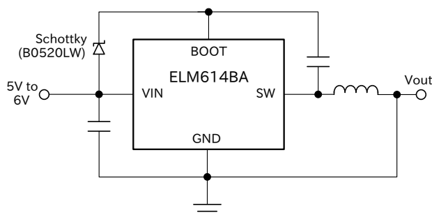
図 3 : V_{\text{in}} \leq 6\text{V} 時の効率向上のためのショットキーダイオードを追加。
