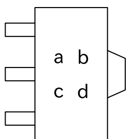
SOT-89
