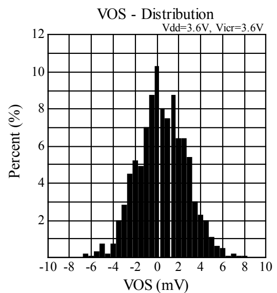
オフセット電圧分布 ( V_{icr}=V_{dd} )
