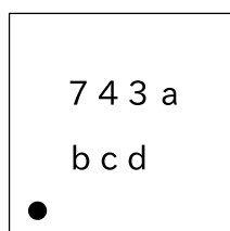
WSON8-2×2
