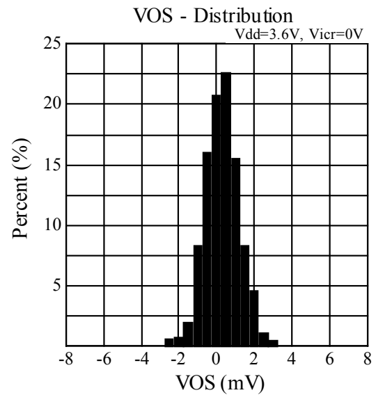
オフセット電圧分布 ( V_{icr}=V_{ss} )
