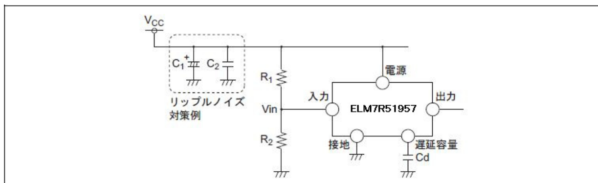
図 6：リップルノイズ対策例
