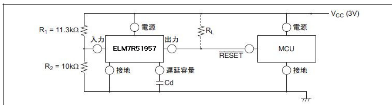
図 2: 3V 系マイコンシステムへの応用例
