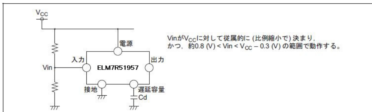
図 7：推奨回路
