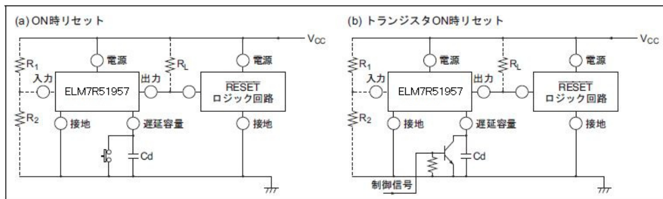
図 3 : ELM7R51957BxBで 電源電圧以外に他のリセット信号を用いる場合
