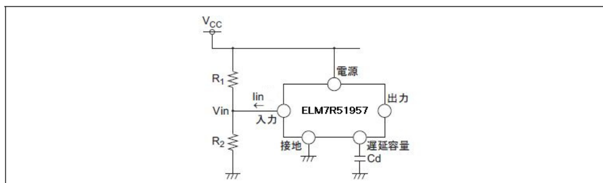
図 9 : 入力電流について
