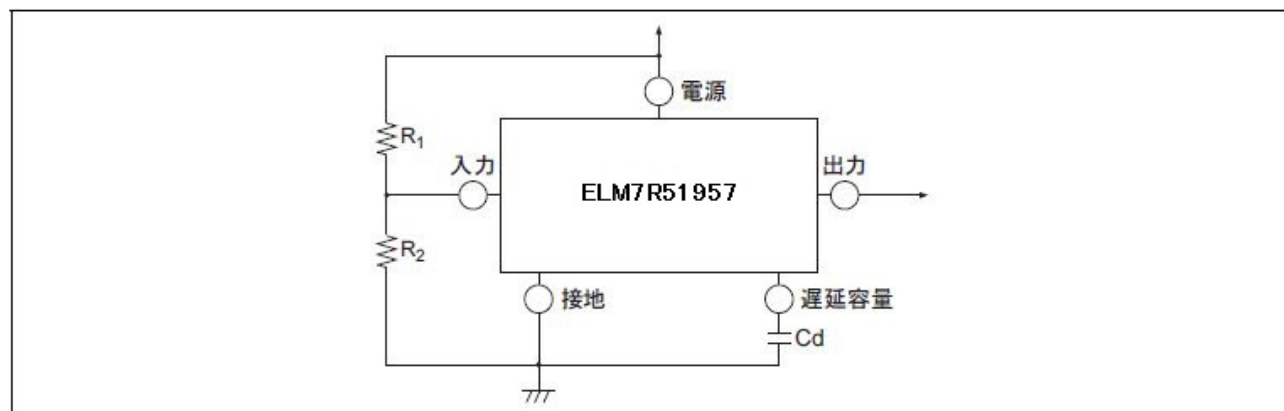
図 4 : 遅延波形発生回路
