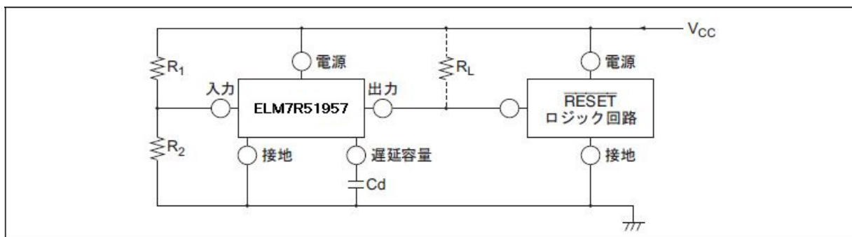
図 1: ELM7R51957 のリセット回路への応用
