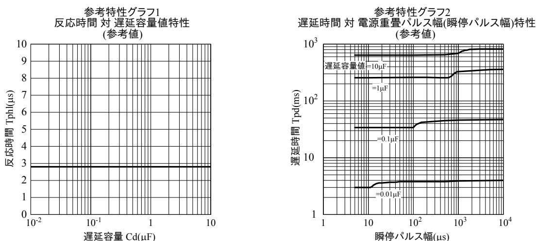
図 11：特性グラフ
