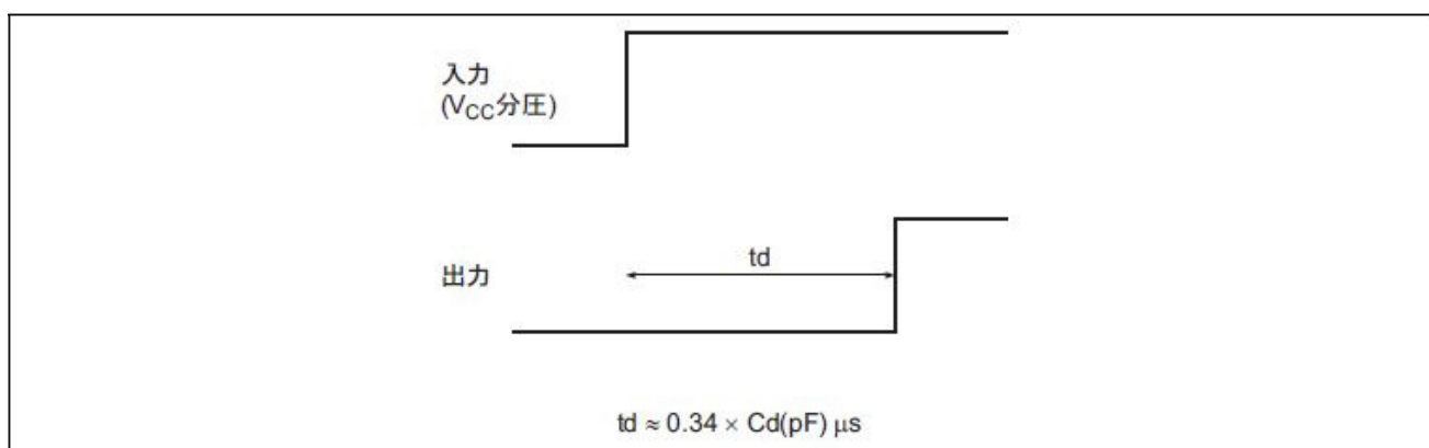
図 5 : 動作波形
