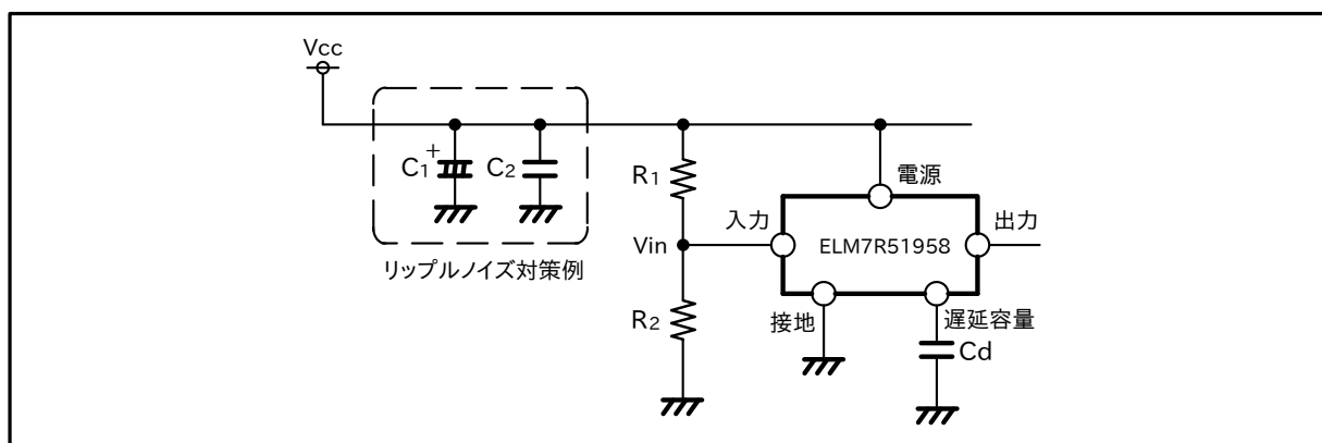
図 6：リップルノイズ対策例
