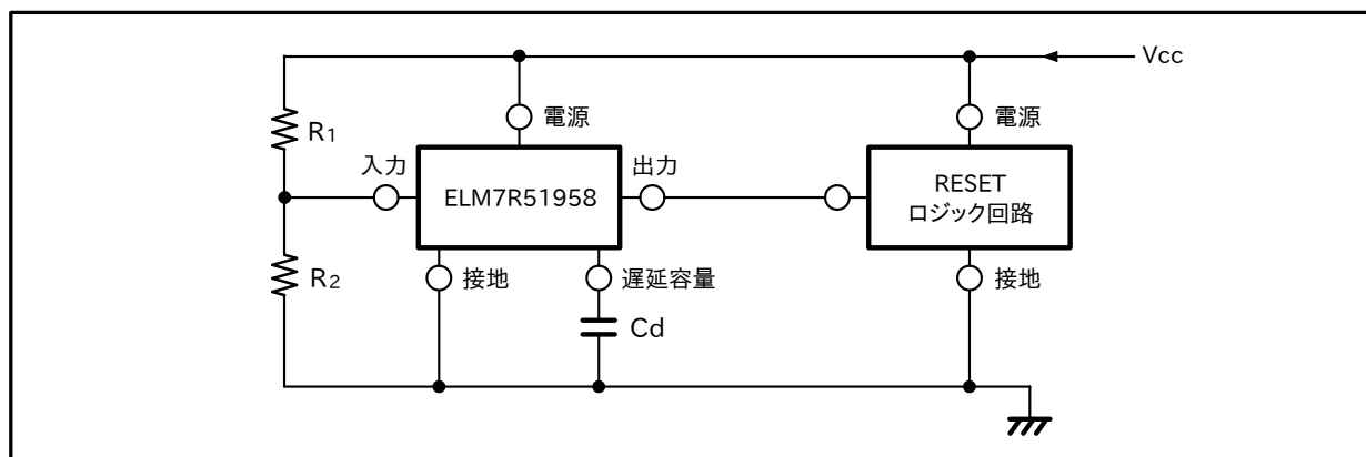
図 1: ELM7R51958 のリセット回路への応用
