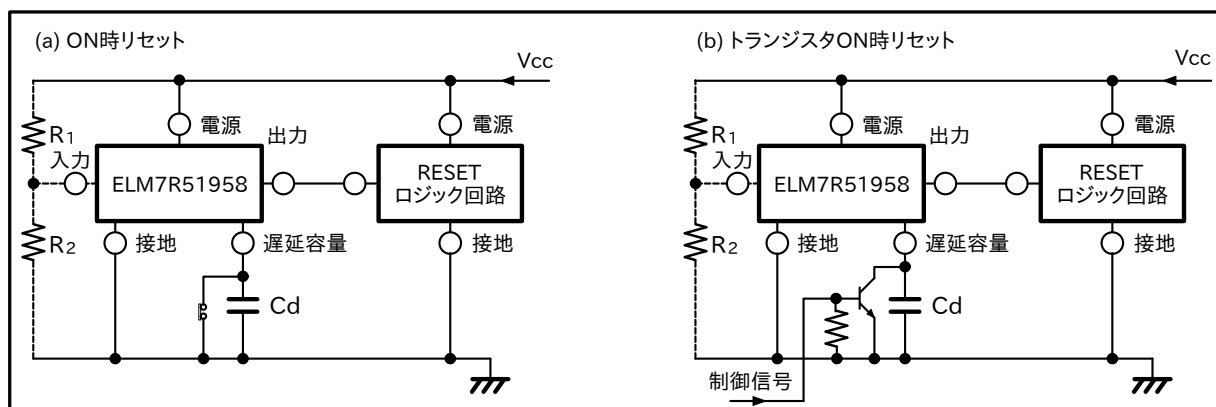
図 3 : ELM7R51958AxBで 電源電圧以外に他のリセット信号を用いる場合
