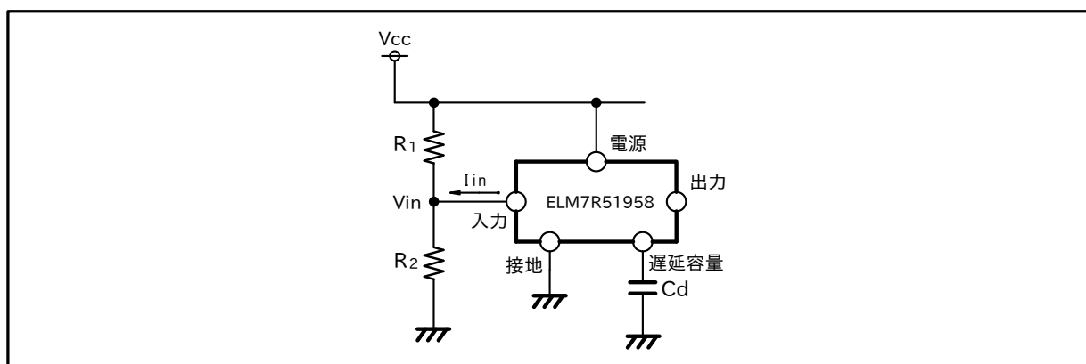
図 9：入力電流について
