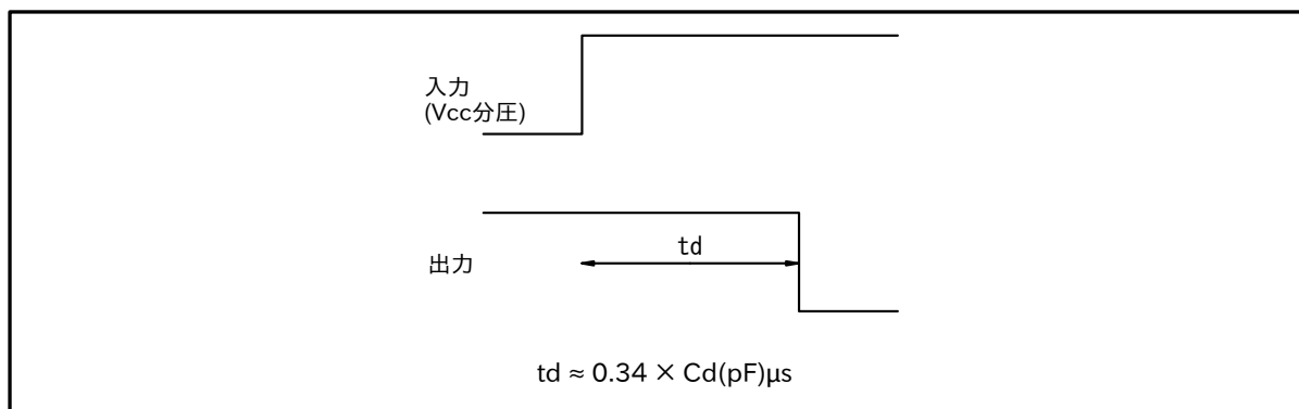
図 5 : 動作波形
