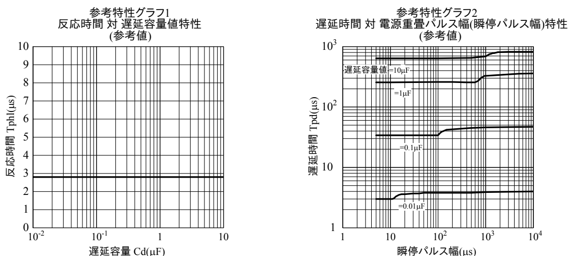
図 11：特性グラフ
