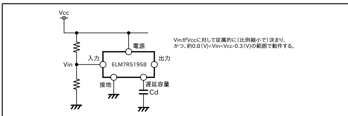
図 7：推奨回路
