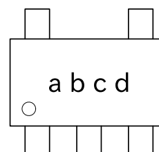
SOT-25
