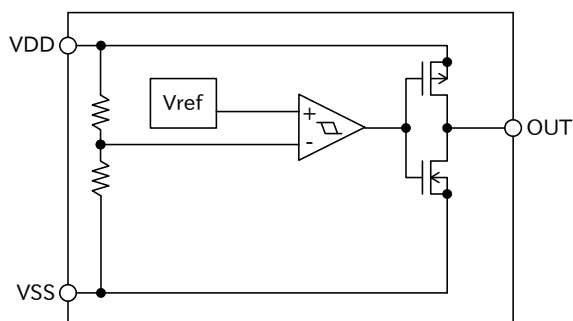
CMOS 出力
