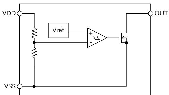
N-ch 出力
