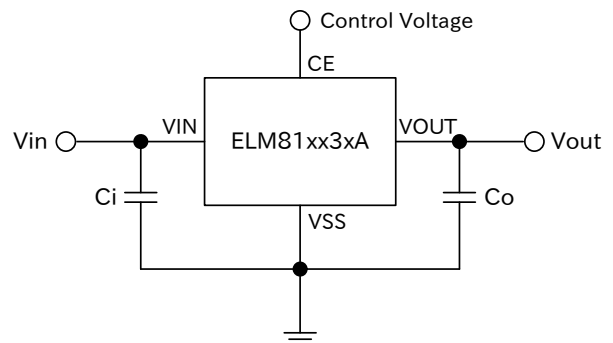
ELM81xx3xA
