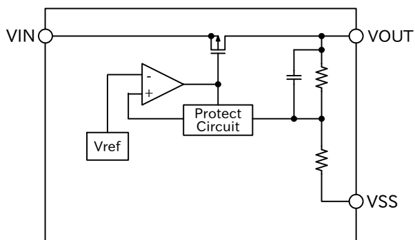
ELM81xxxA
