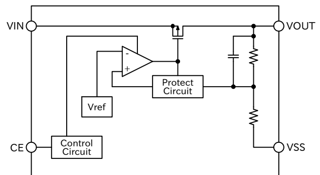
ELM81xx3xA
