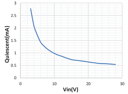
Steady State Test (Buck)
