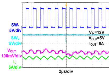
Steady State Test (Buck)
