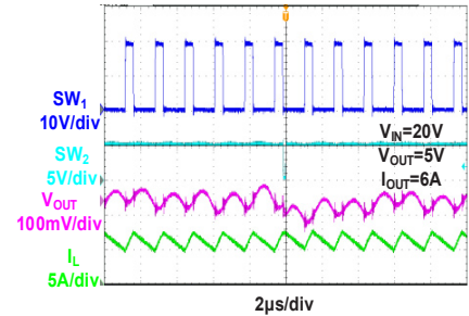
Steady State Test (Buck)
