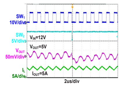
Steady State Test (Buck)
