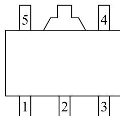
SOT-89-5(俯视图)
