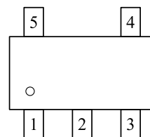
SOT-25(俯视图)
