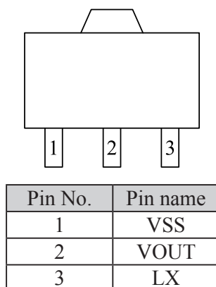
SOT-89(TOP VIEW)
