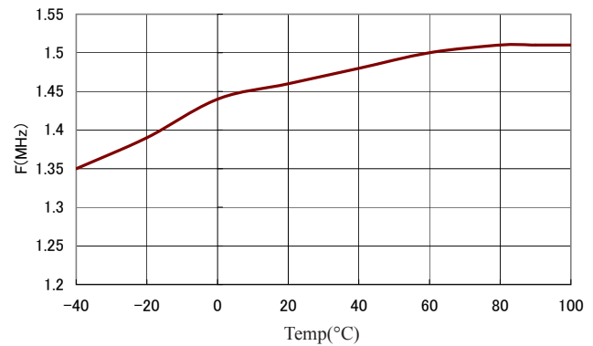
Temp-F
