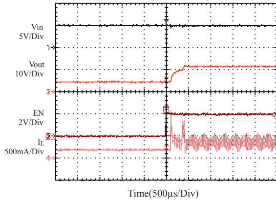
Enable On
