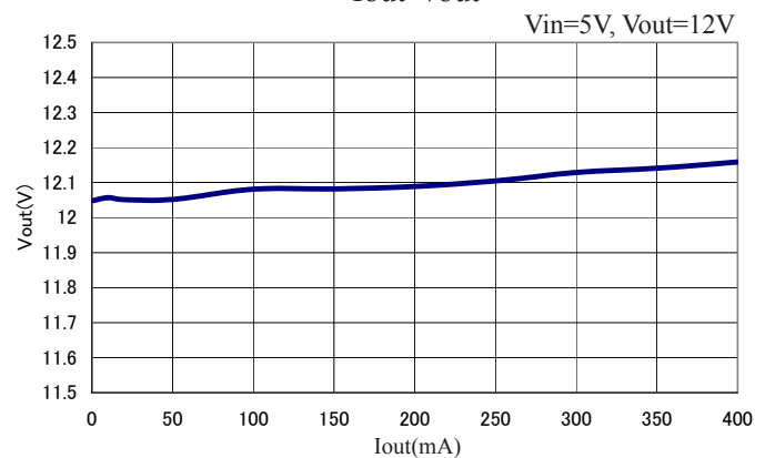
Iout-Vout
