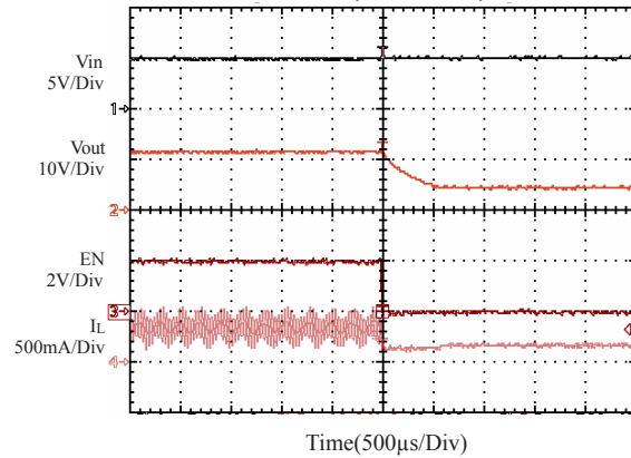
Enable Off
