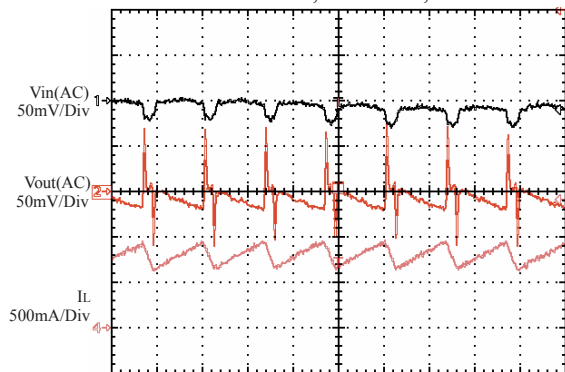
Ripple
